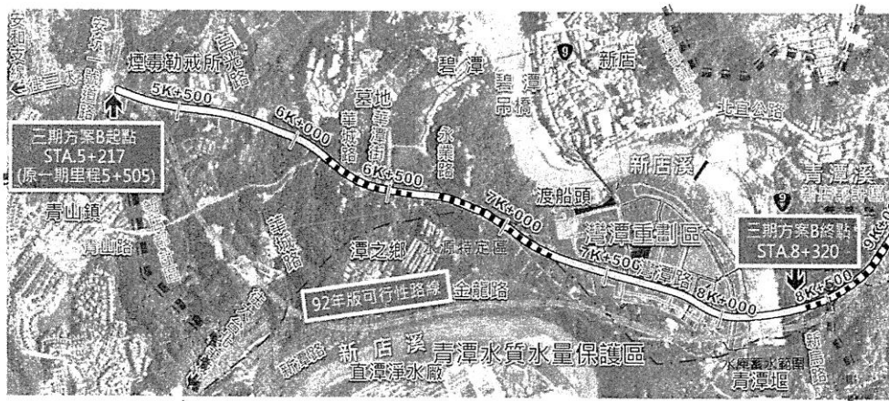
安坑1號道路第三期工程示意圖
